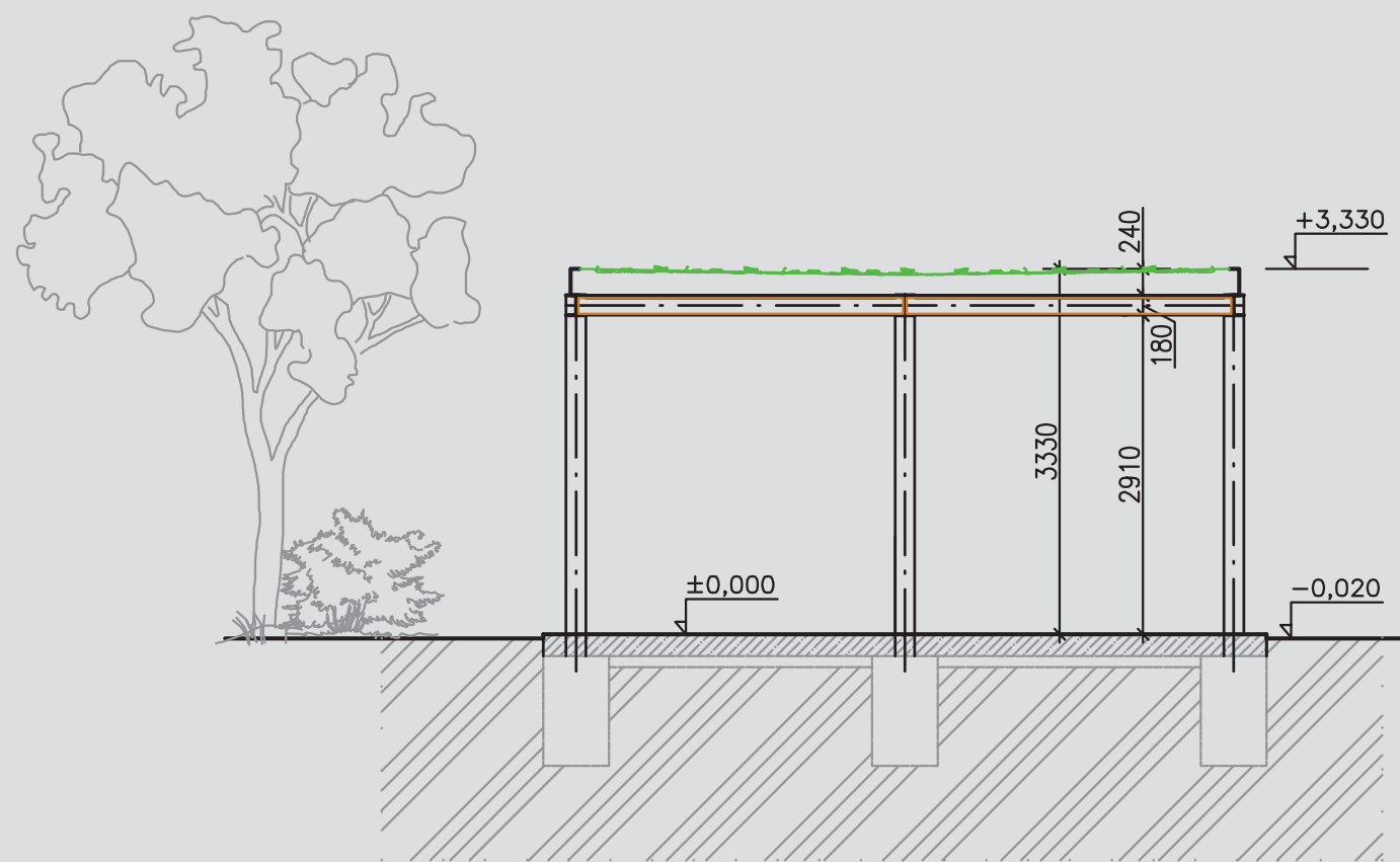
PŘÍČNÝ ŘEZ 2-2
