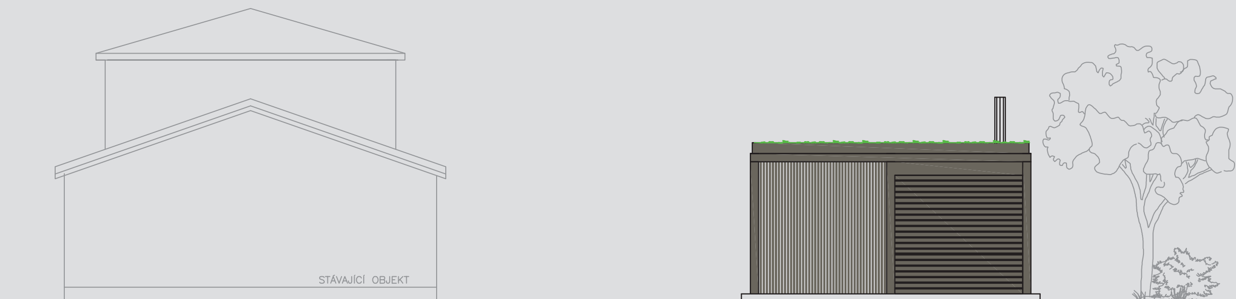
SEVERNÍ POHLED
