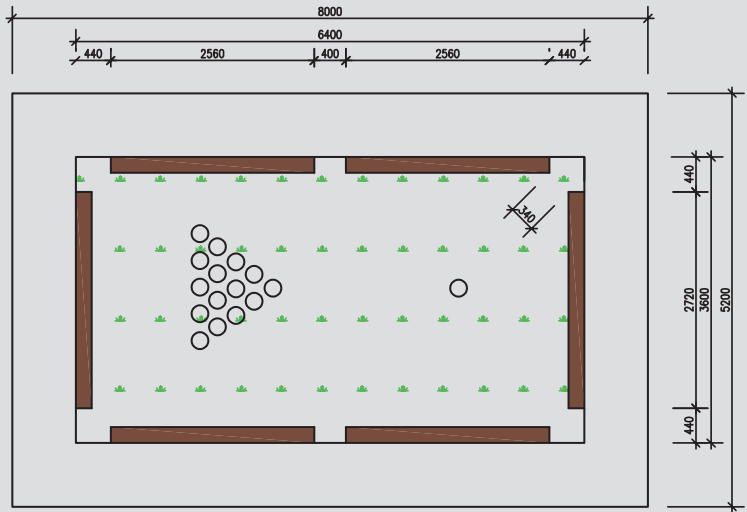
PŮDORYS
