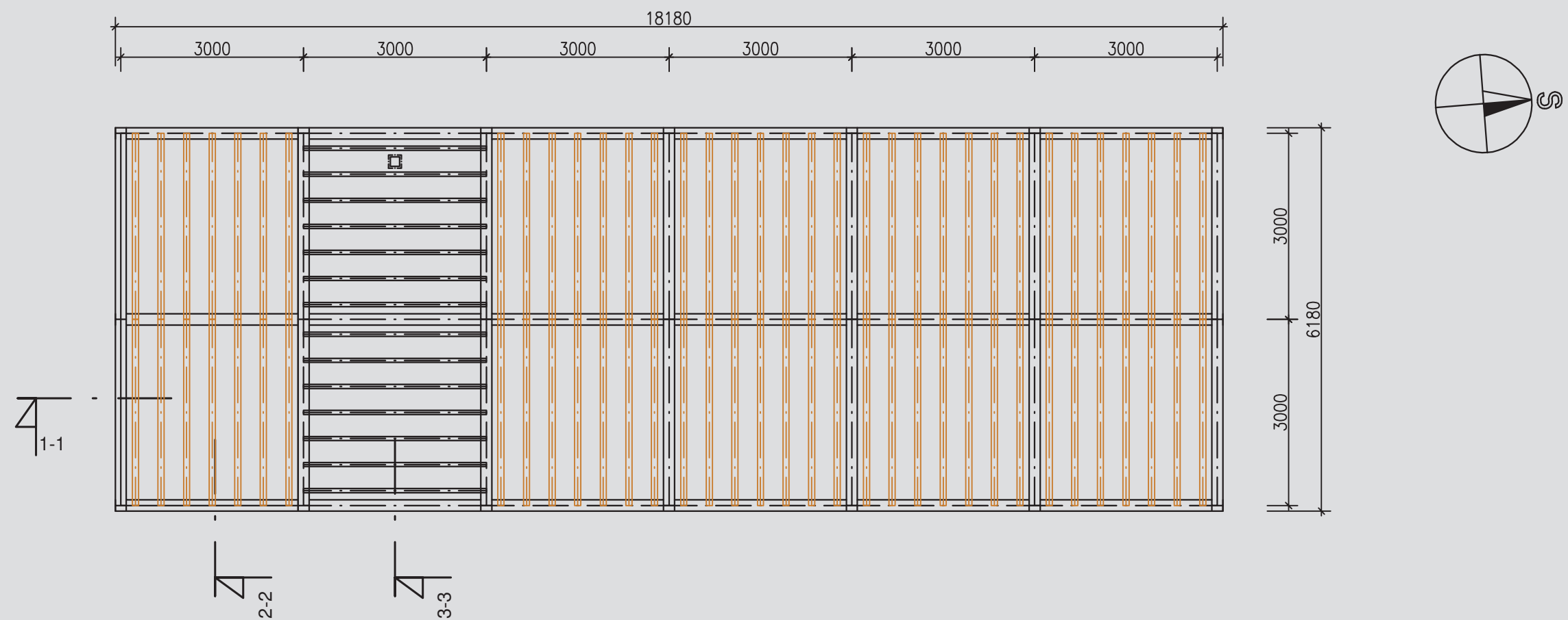
PŮDORYS KONSTRUKCE STROPU
