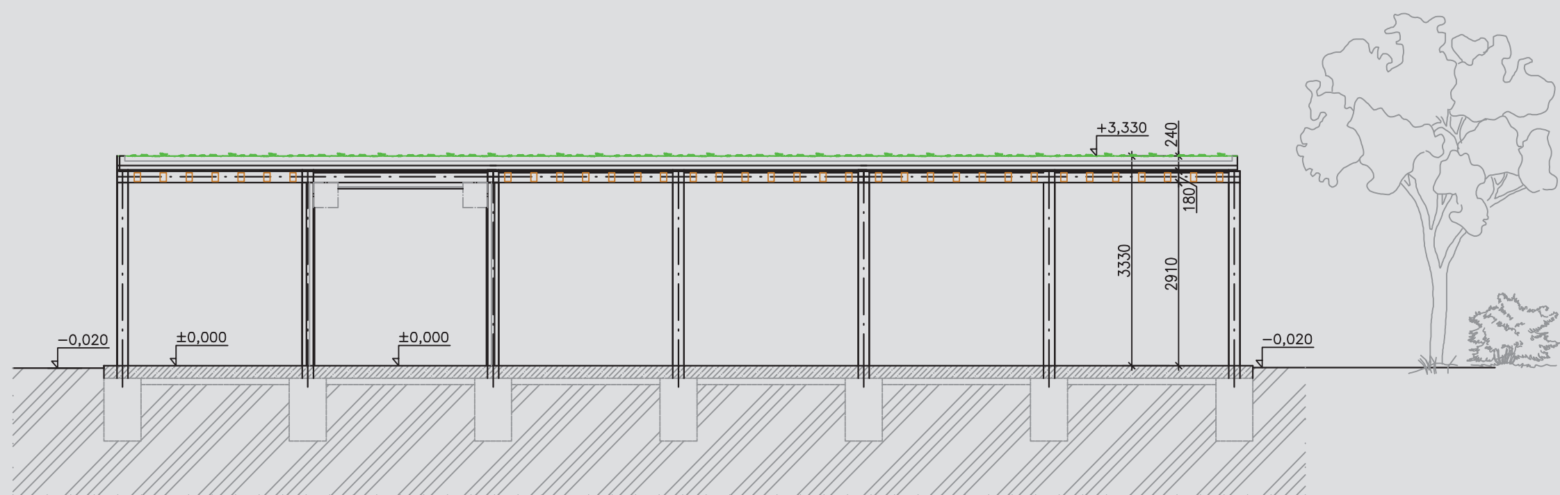
PODÉLNÝ ŘEZ 1-1
